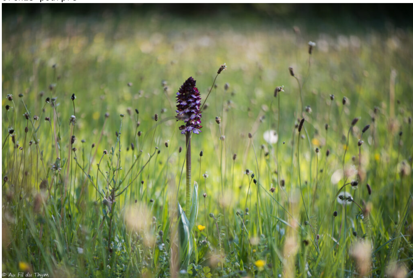
Orchis pourpre
